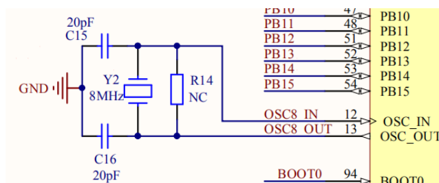
图 2 晶振电路
